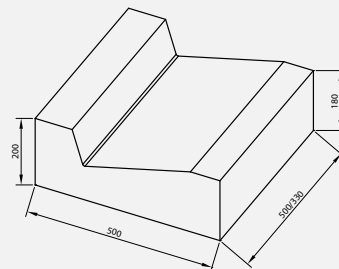
Płyta ściekowa trójkątna
