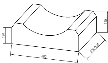
Płyta ściekowa korytkowa
