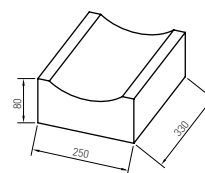
Płyta ściekowa korytkowa/chodnikowa
