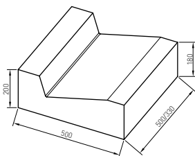
Płyta ściekowa trójkątna
